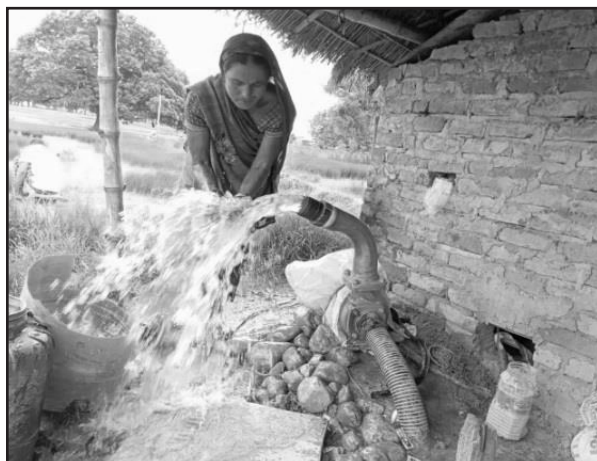
मोटराइज स्यालो टयूवेल जडान पछि धान बालीमा सिचाई गर्दै महिला
